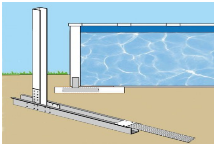
PRESJEK SAMONOSIVE KONSTRUKCIJE SA NOSAČIMA POD BAZENOM
